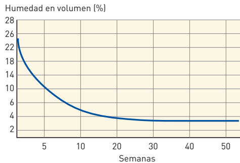
Curva de secado de los bloques de hormigón celular YTONG de 20 cm de espesor en temperatura ambiente interior
