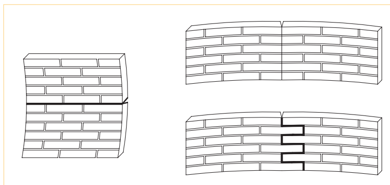
Plano de rotura paralelo a los tendeles (flexión vertical)
