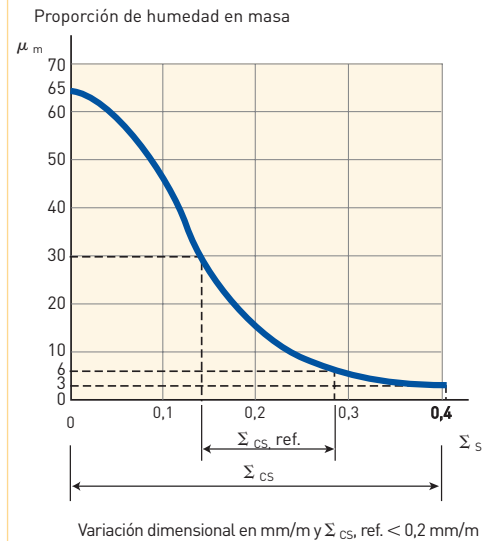
Retracción debida al secado del hormigón celular YTONG
