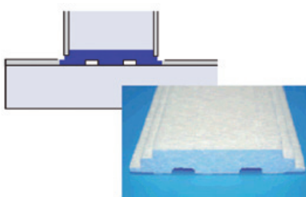
Bandas elásticas de porexpan escalonadas
