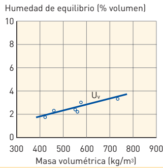
Proporción de humedad de equilibrio (en volumen) en función de la masa volumétrica
