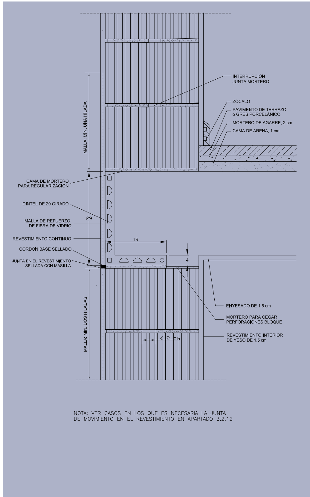
Figura 38: Apoyo del forjado en muro portante. Solución con pieza L girada.
