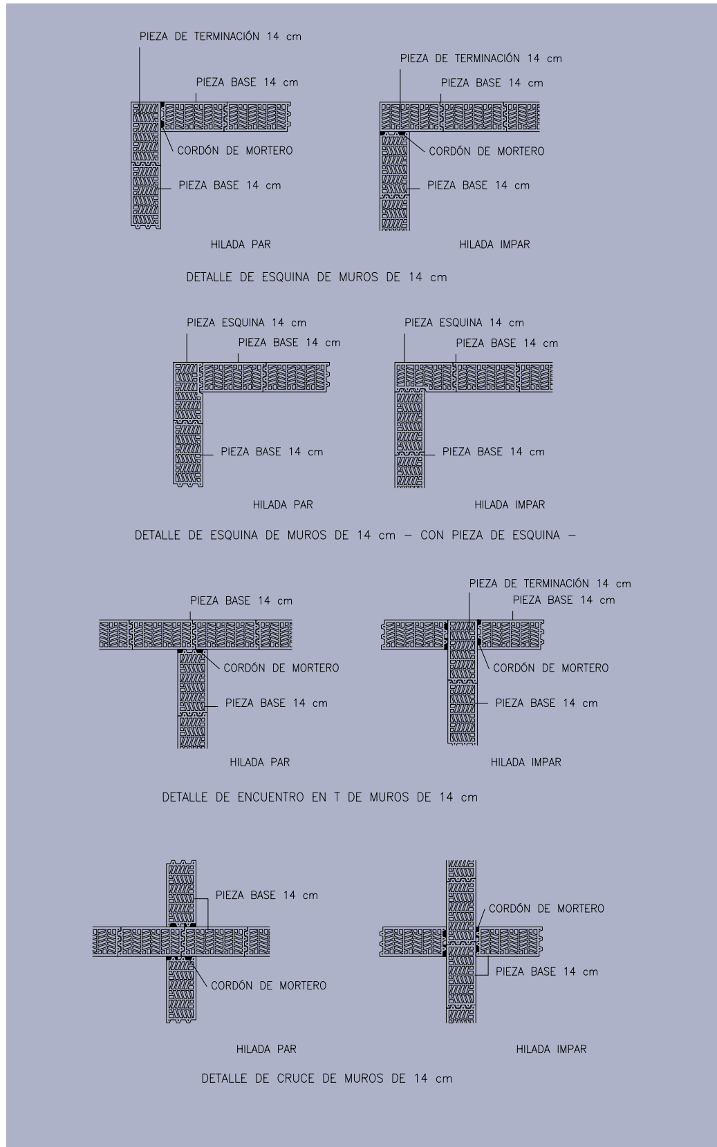
Figura 20: Detalles de encuentro con piezas de 14 cm.
