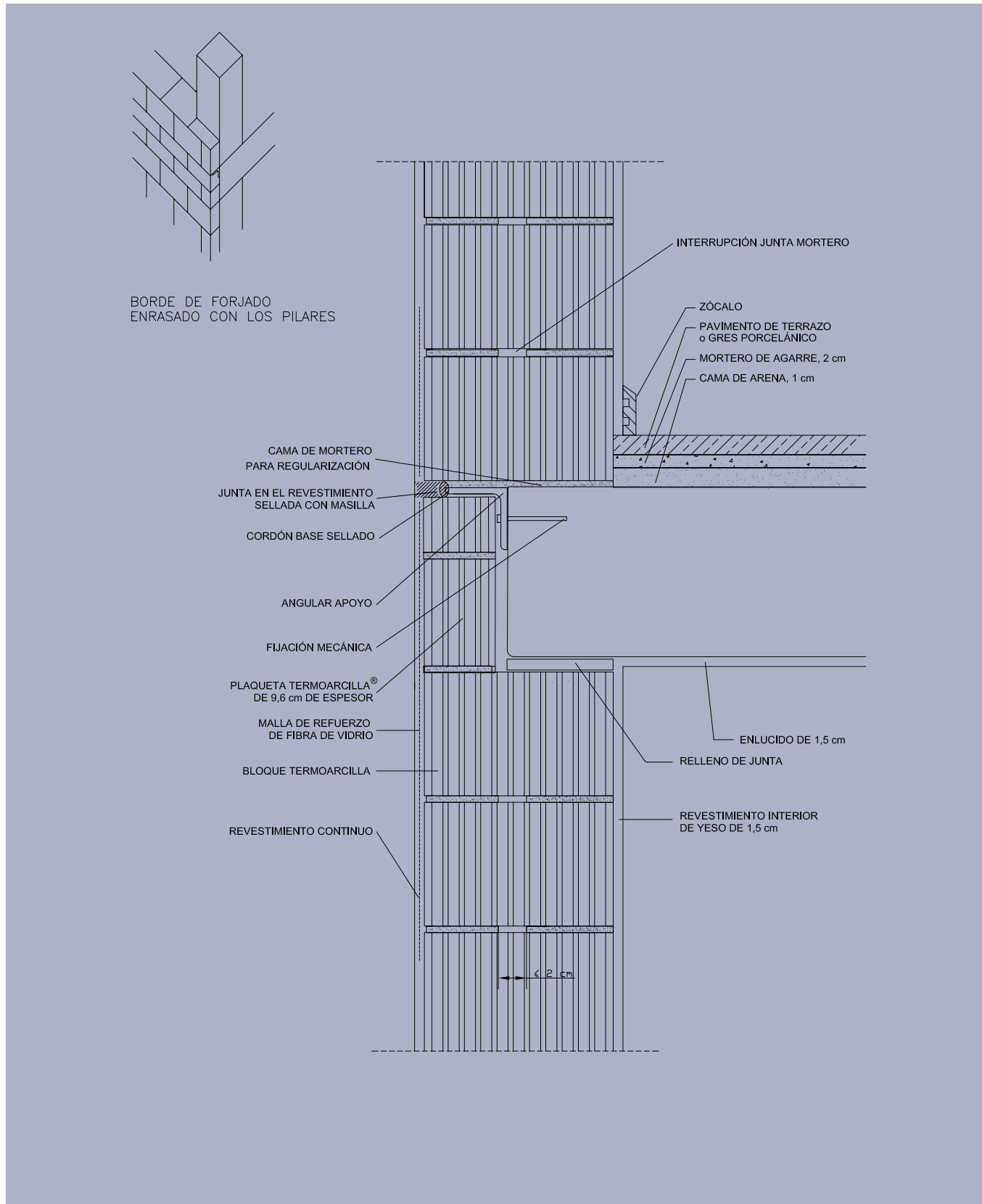
Figura 43: Encuentro con el forjado. Variante con perfil.
