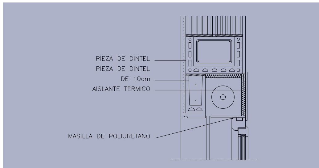
Figura 29: Dintel con caja de persiana.
