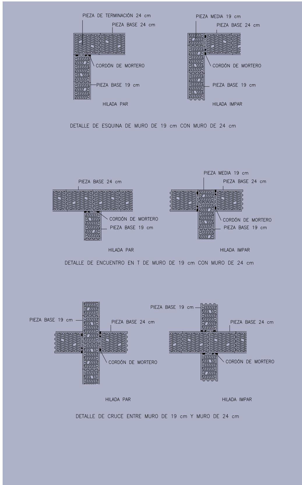
Figura 18: Detalles de encuentro de piezas de 19 cm con piezas de 24 cm.
