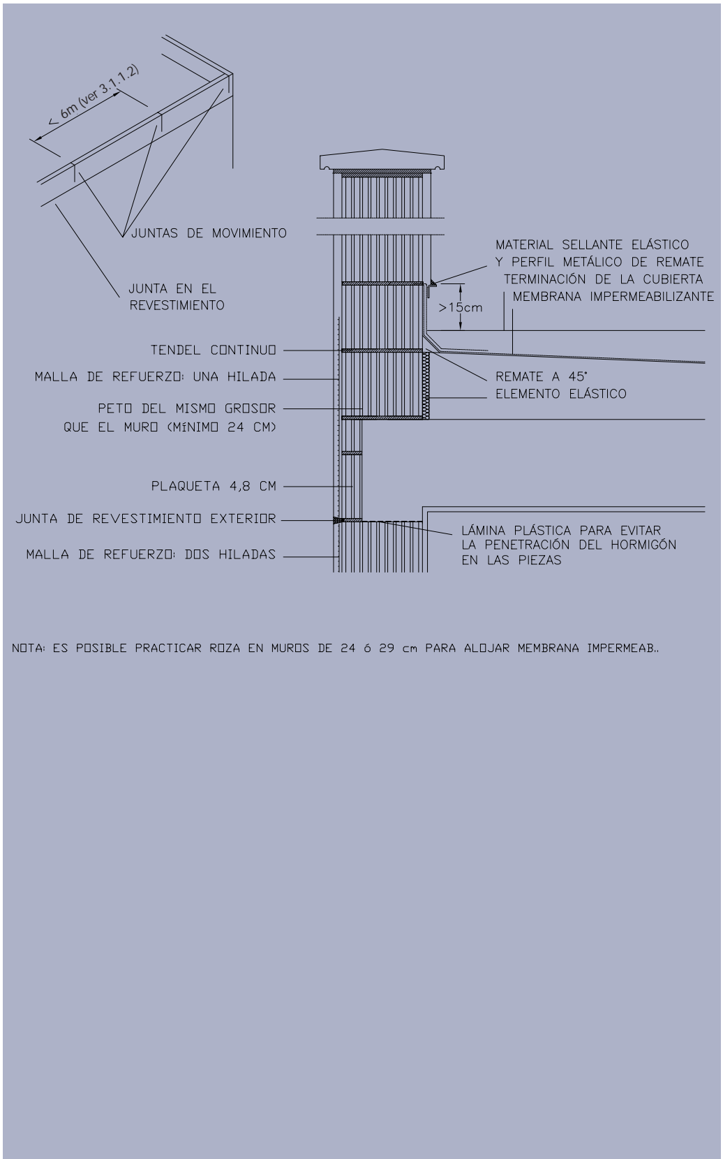
Figura 40: Apoyo del último forjado en caso de azotea.
