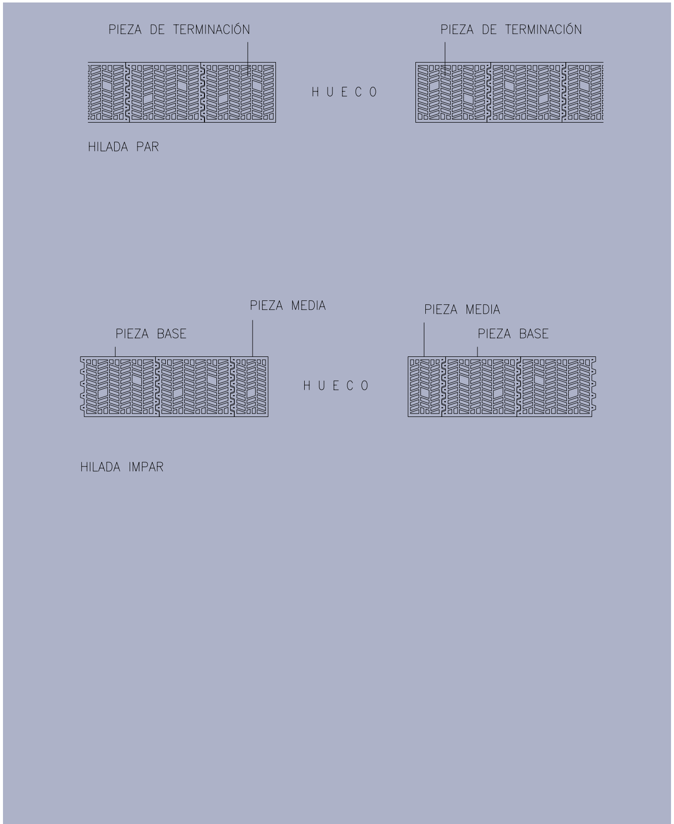
Figura 50: Ejecución de las jambas.
