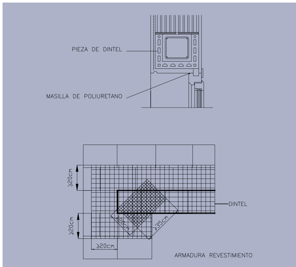
Figura 28: Dintel sin caja de persiana.
