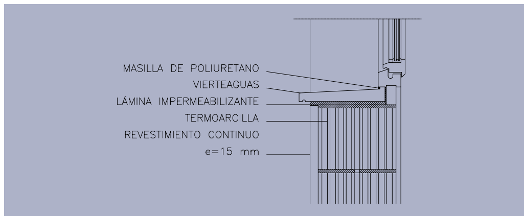
Figura 32: Antepecho y alféizar.
