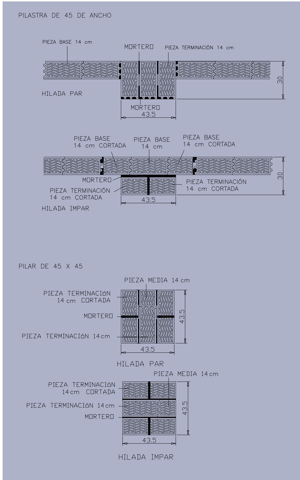
Figura 7: Pilastra de 45 cm de ancho y pilar de 45x45 cm.
