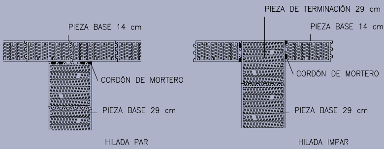
DETALLE DE ENCUENTRO EN T DE MURO DE 14 cm CON MURO DE 29 cm
