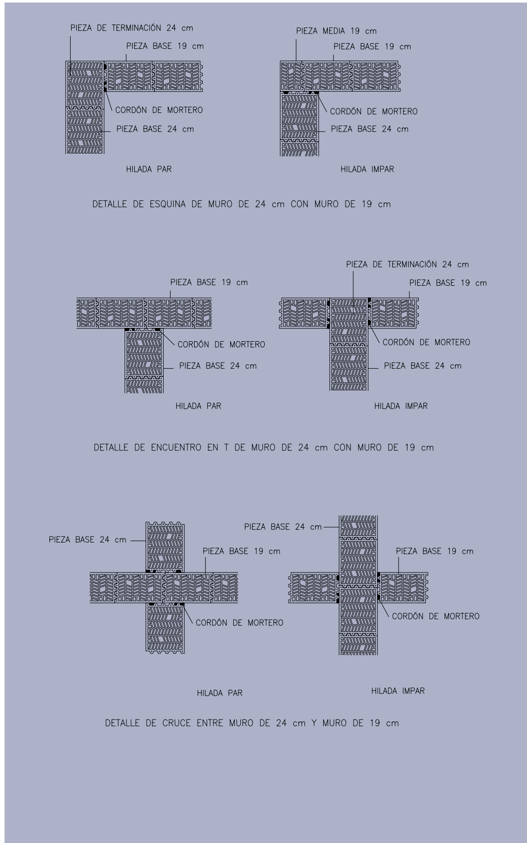
Figura 14: Detalles de encuentro de piezas de 24 cm con piezas de 19 cm.
