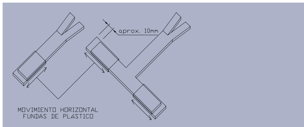
Figura 4: Llaves para juntas de movimiento.
