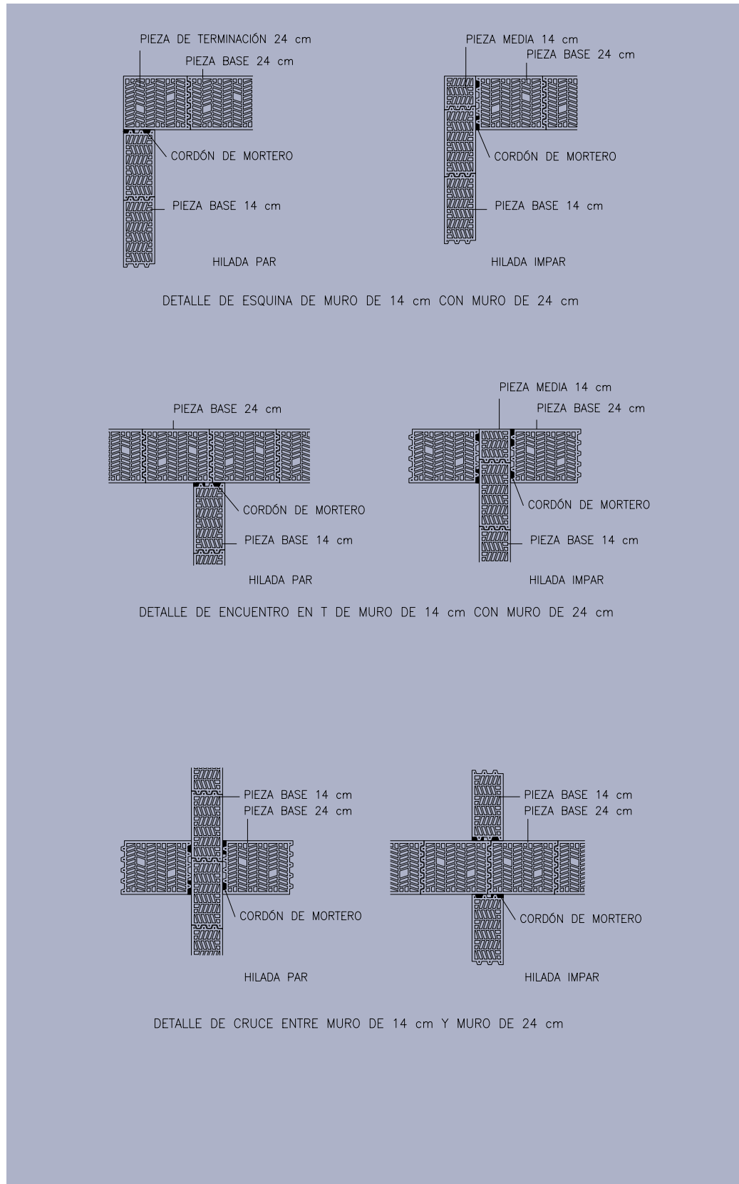
Figura 22: Detalles de encuentro de piezas de 14 cm con piezas de 24 cm.
