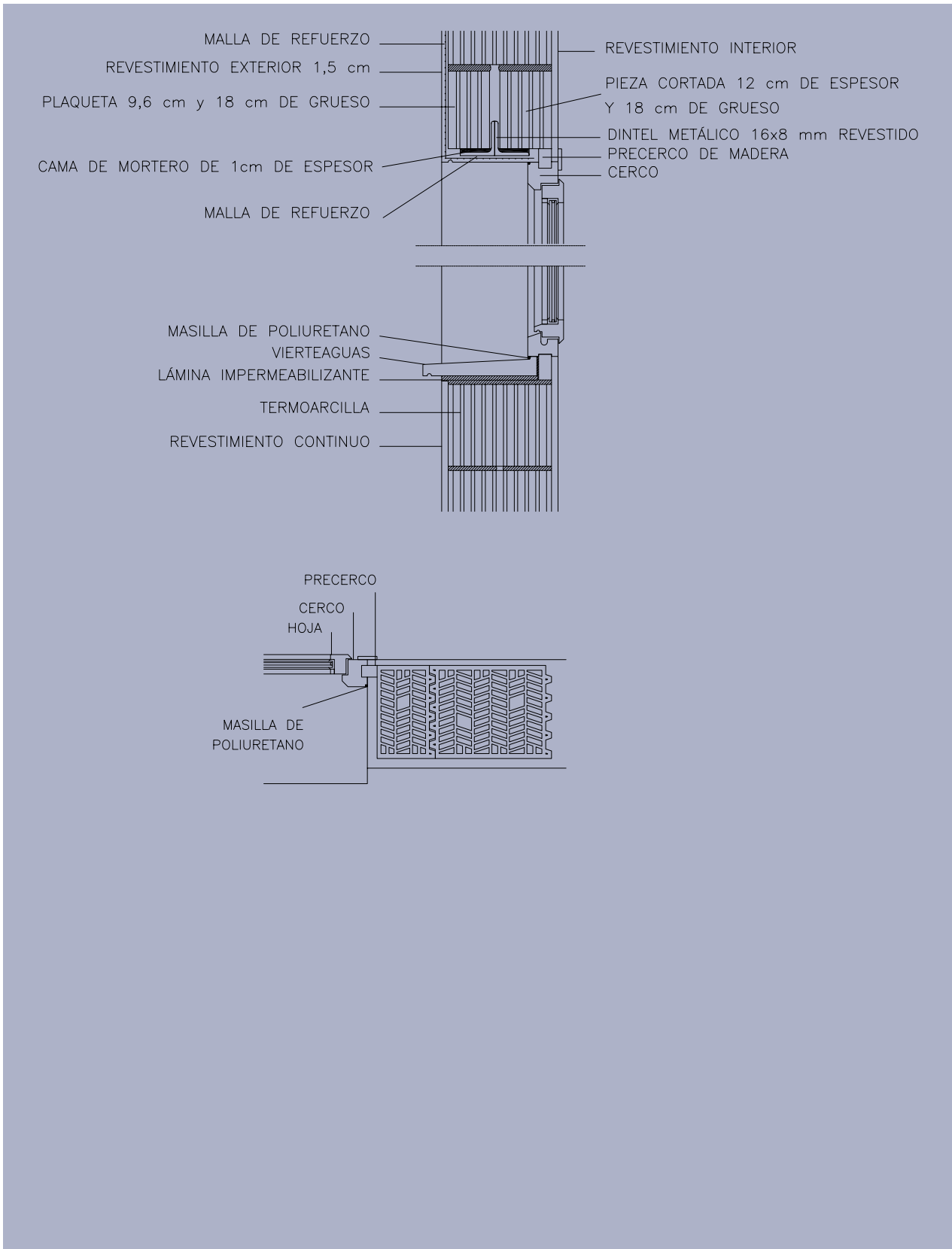
Figura 35: Huevo de ventana. Solución de dintel con perfil metálico en T en muro de 24 cm, sin caja de persiana.
