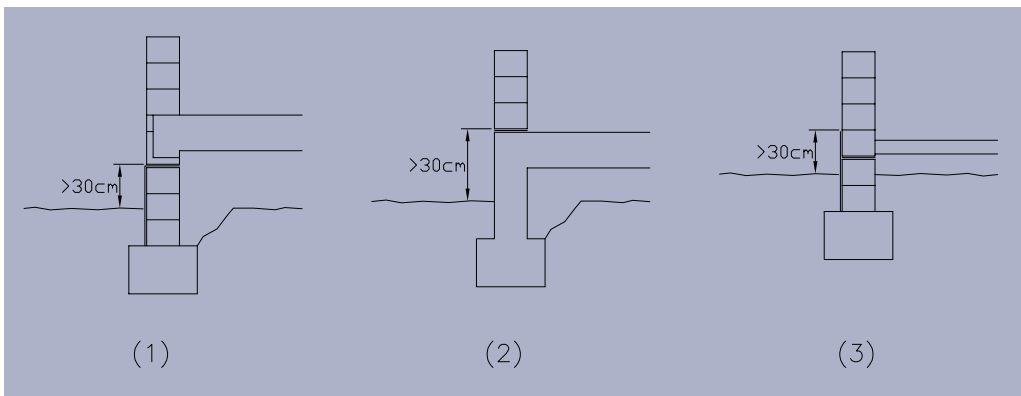
Figura 26: Arranque de fachadas. Esquemas.
