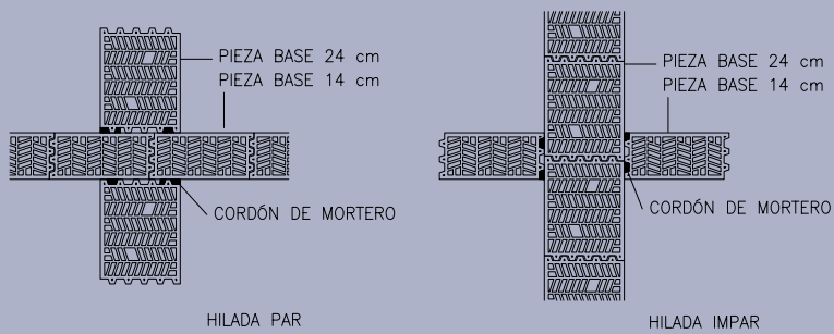
DETALLE DE CRUCE ENTRE MURO DE 24 cm Y MURO DE 14 cm
