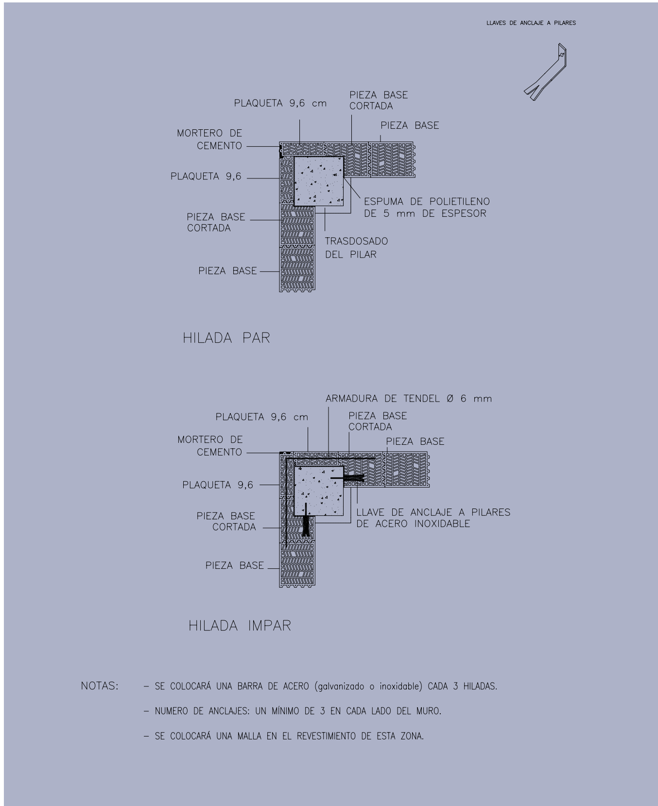
Figura 46: Unión entre muros de cerramiento y soportes en esquina.
