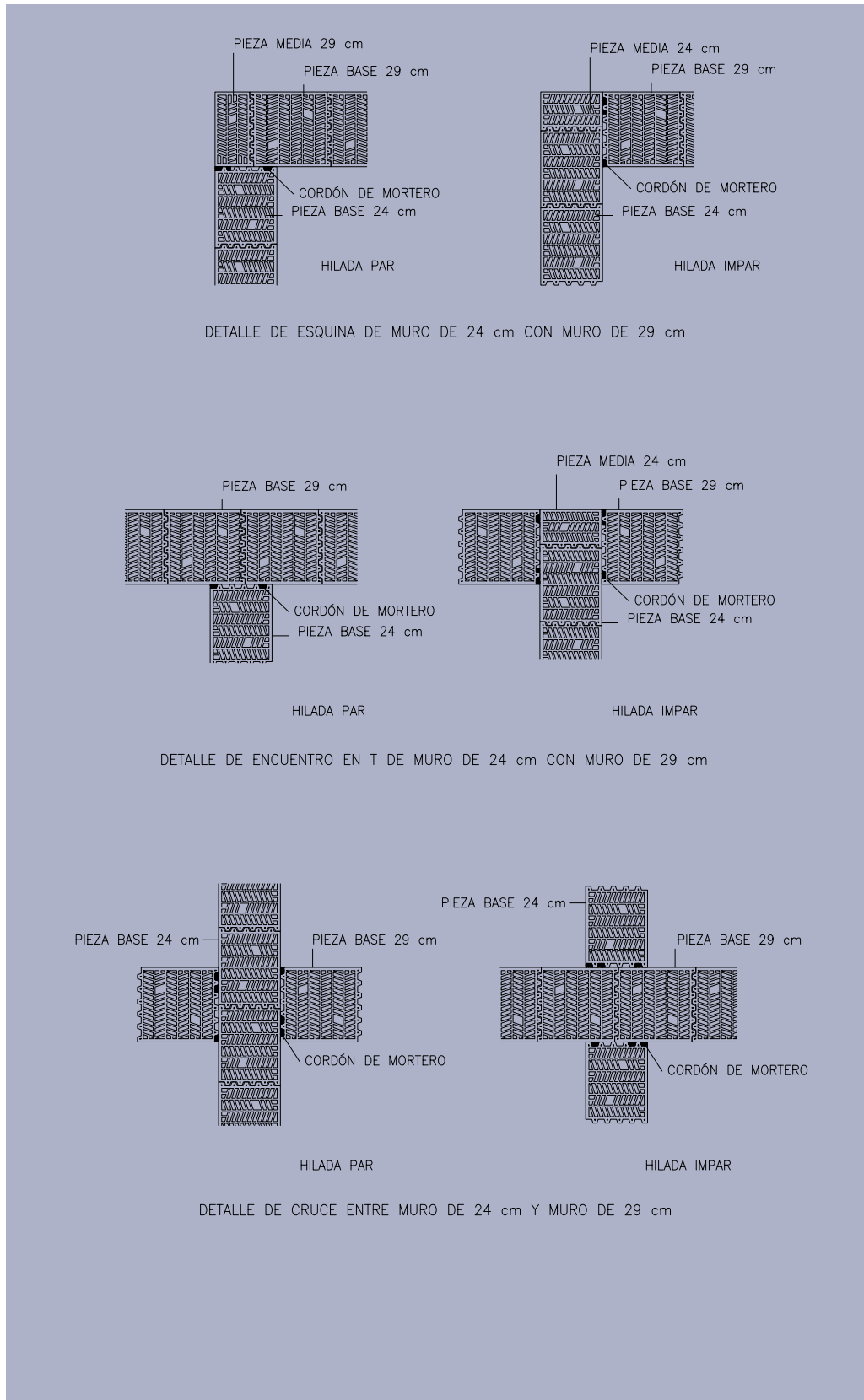
Figura 13: Detalles de encuentro de piezas de 24 cm con piezas de 29 cm..
