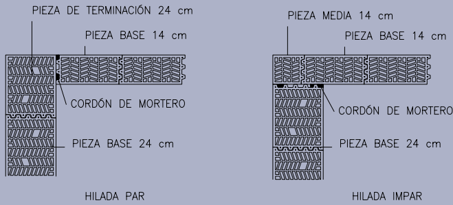
DETALLE DE ESQUINA DE MURO DE 24 cm CON MURO DE 14 cm
