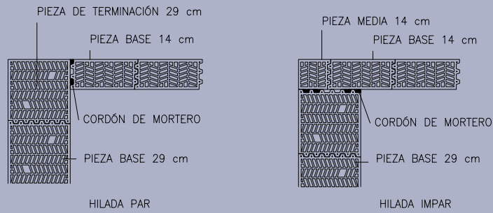
DETALLE DE ESQUINA DE MURO DE 29 cm CON MURO DE 14 cm
