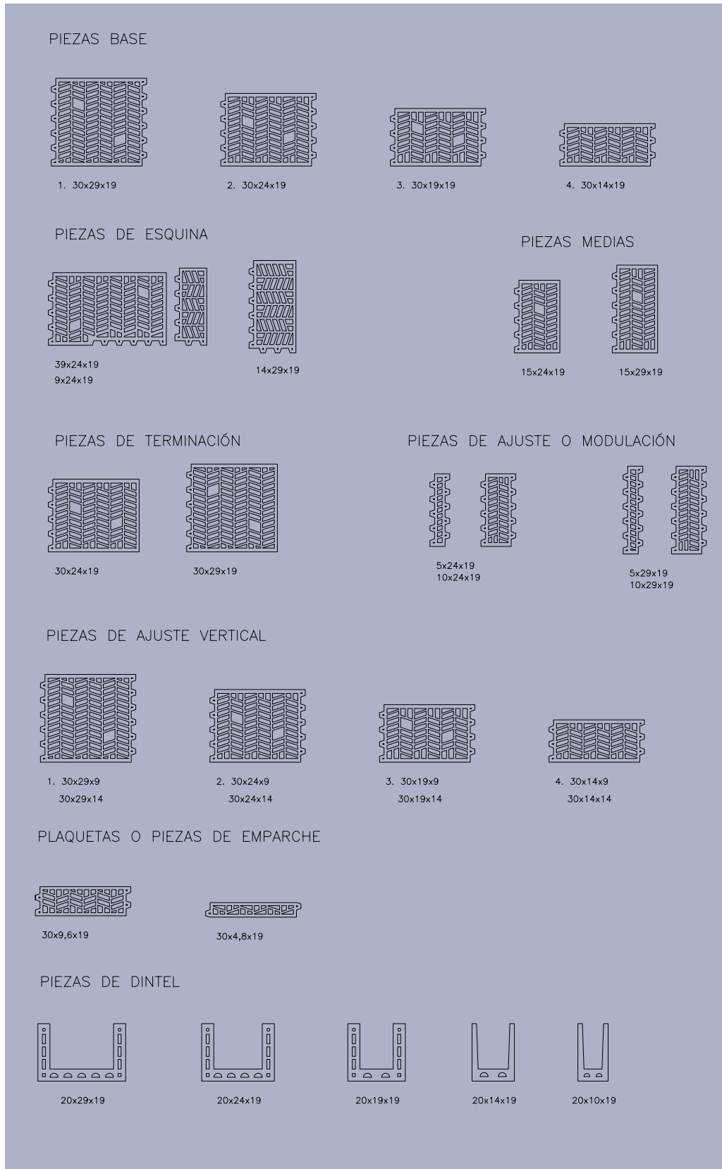
Figura 1: Piezas del sistema.
