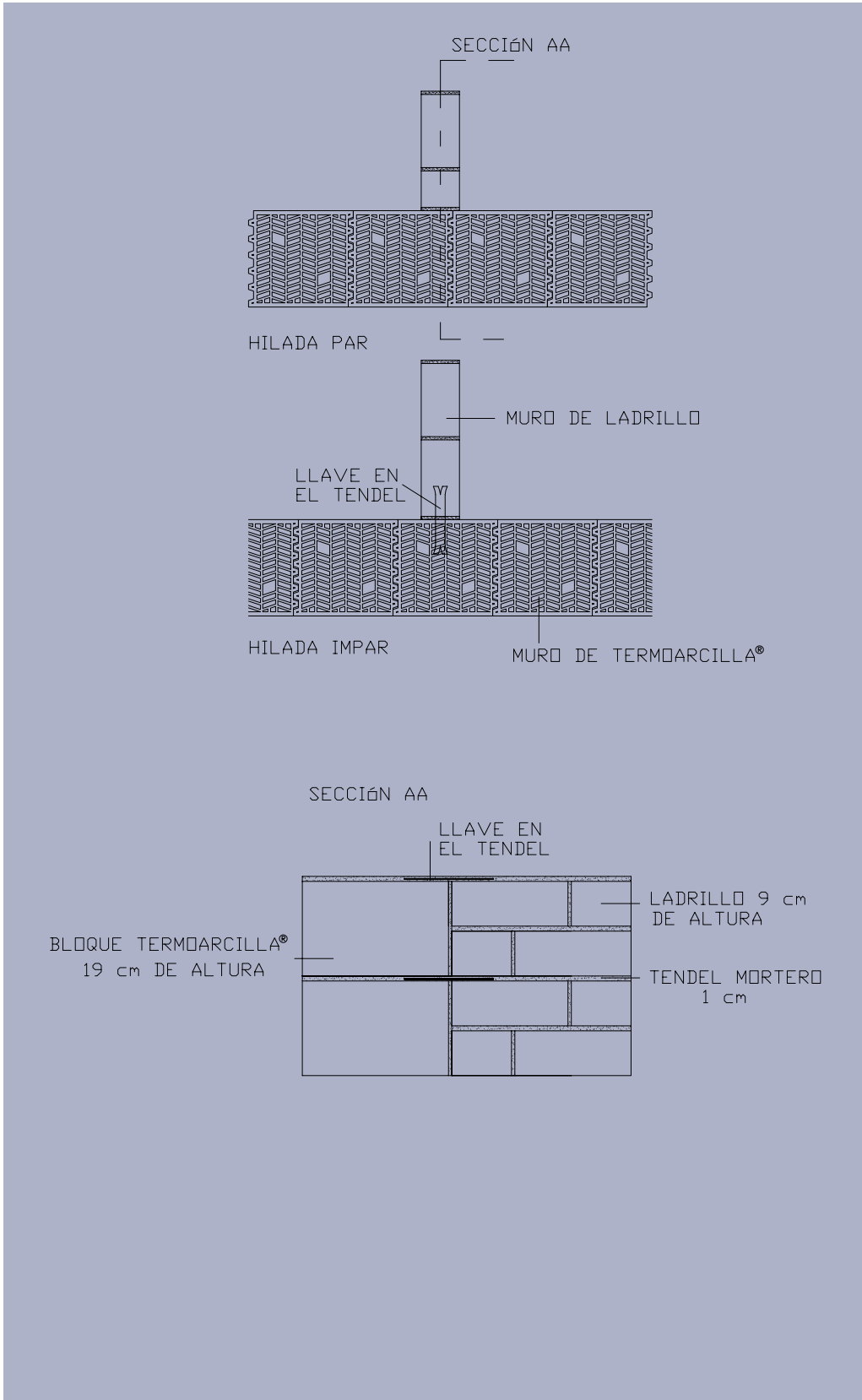
Figura 6: Enlace de muro de ladrillo con muro de Termocilla®.
