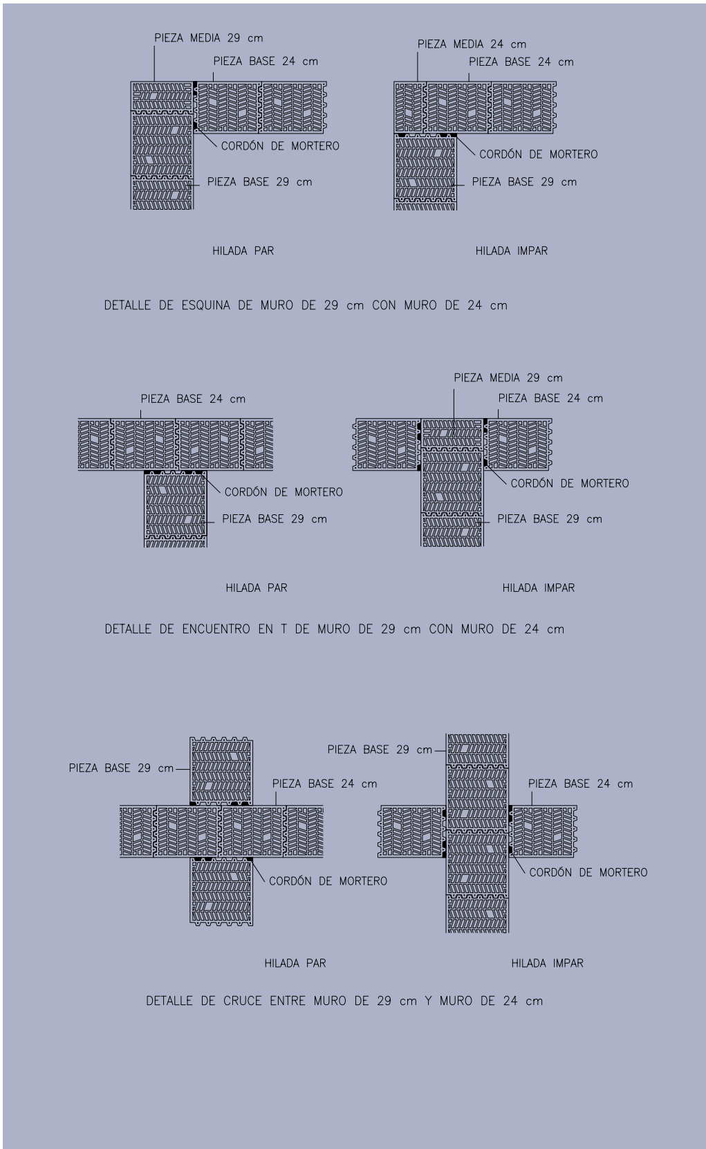
Figura 9: Detalles de encuentro de piezas de 29 cm con piezas de 24 cm.
