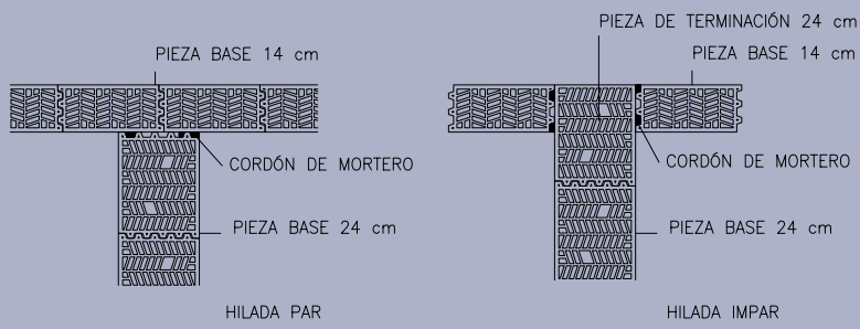
DETALLE DE ENCUENTRO EN T DE MURO DE 24 cm CON MURO DE 14 cm
