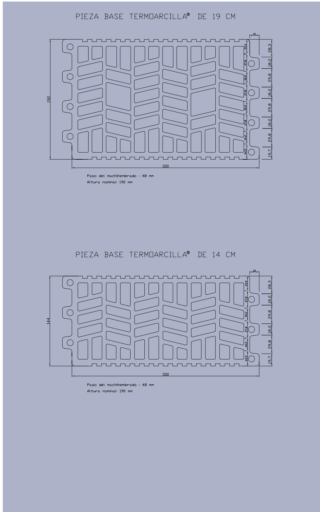
Figura 3: Piezas base de 19 y 14 cm.
