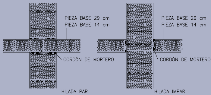
DETALLE DE CRUCE ENTRE MURO DE 29 cm Y MURO DE 14 cm
