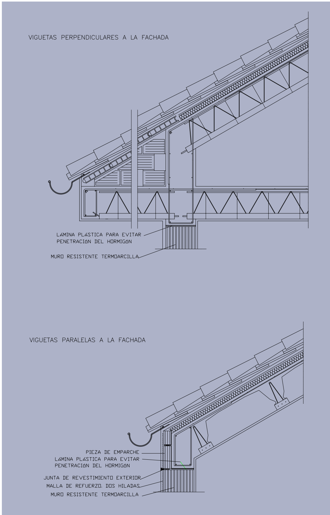
Figura 41: Apoyo del último forjado en caso de tejado.
