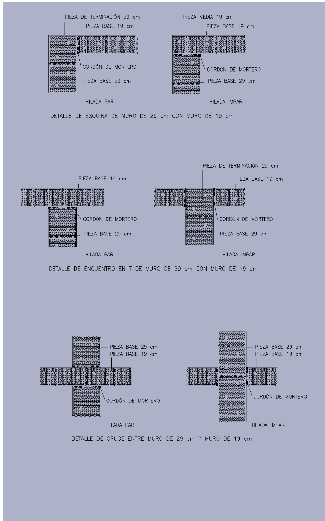
Figura 10: Detalles de encuentro de piezas de 29 cm con piezas de 19 cm.
