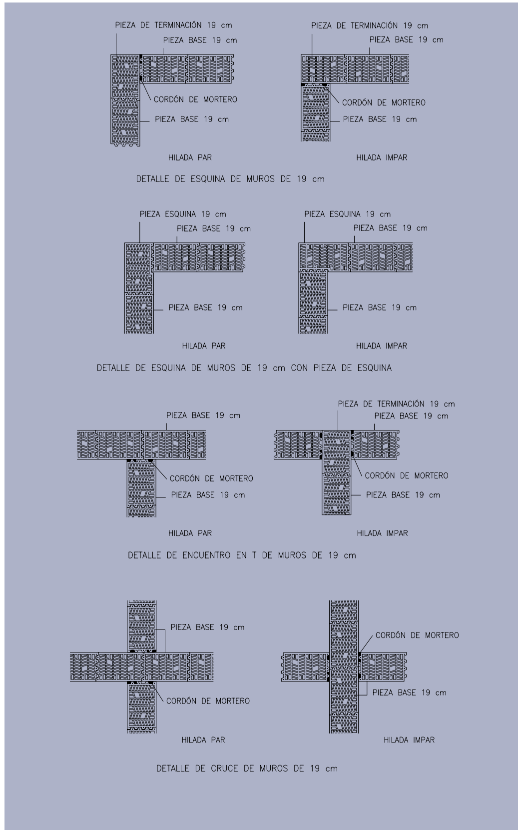
Figura 16: Detalles de encuentro con piezas de 19 cm.
