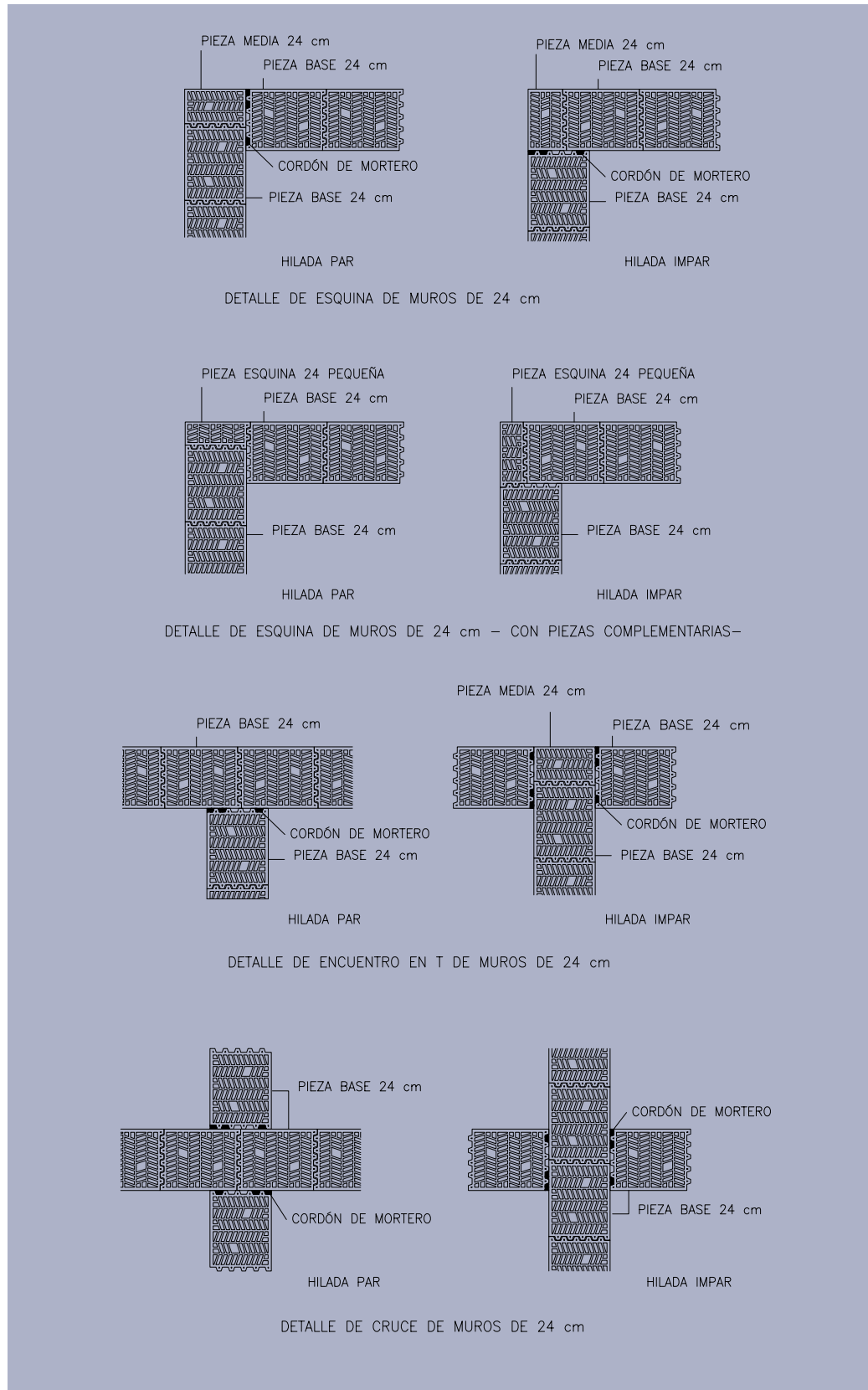
Figura 12: Detalles de encuentro con piezas de 24 cm.
