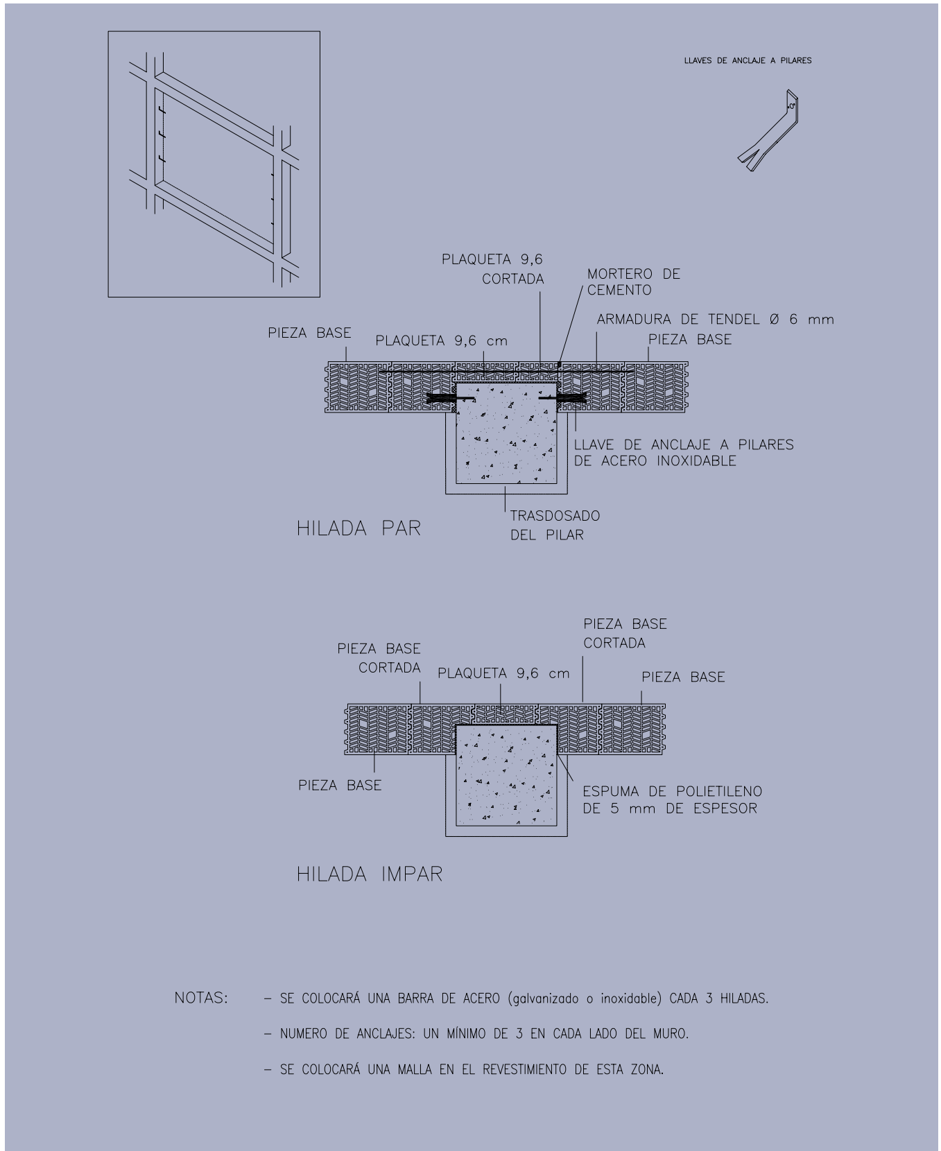
Figura 45: Unión entre muros de cerramiento y soportes con ancho mayor de 30 cm.
