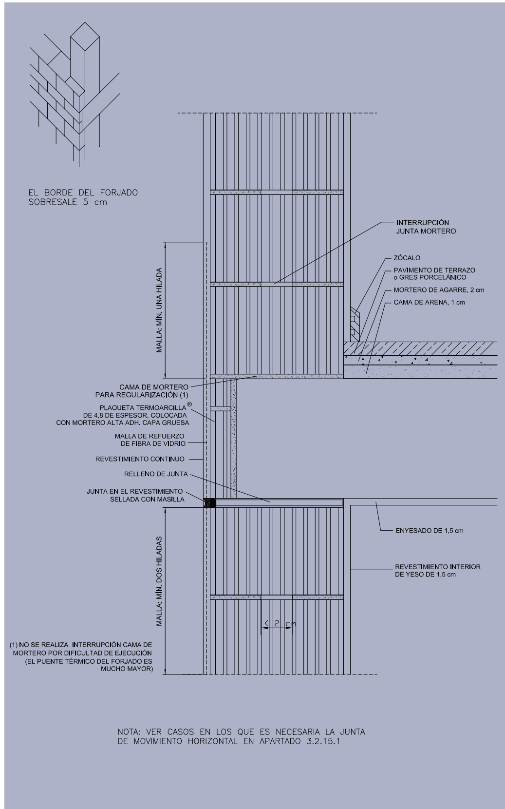
Figura 42: Encuentro con el forjado.
