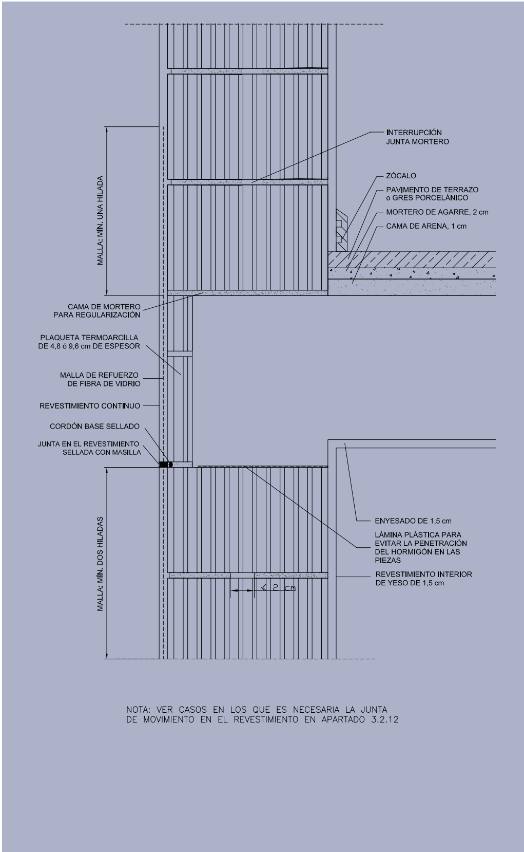
Figura 37: Apoyo del forjado en muro portante. Solución con plaqueta.
