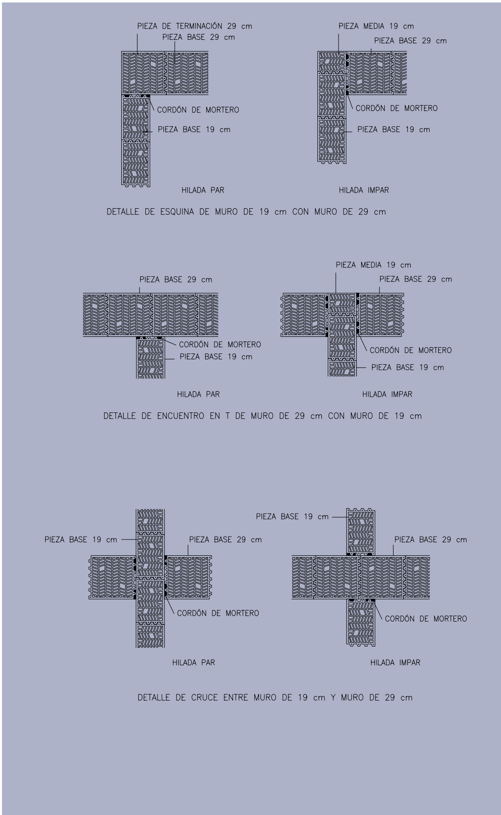
Figura 17: Detalles de encuentro de piezas de 19 cm con piezas de 29 cm.
