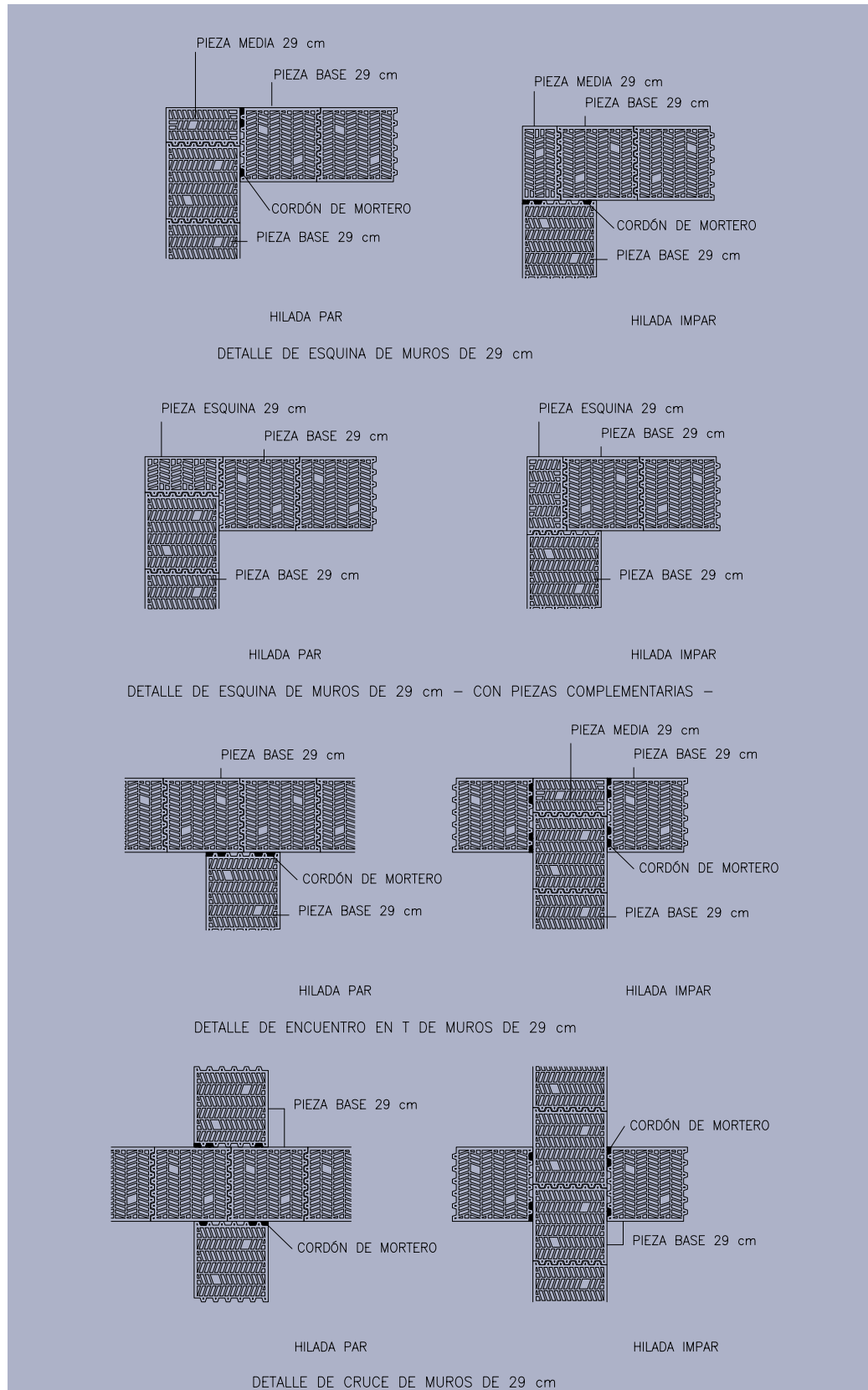
Figura 8: Detalles de encuentro con piezas de 29 cm.
