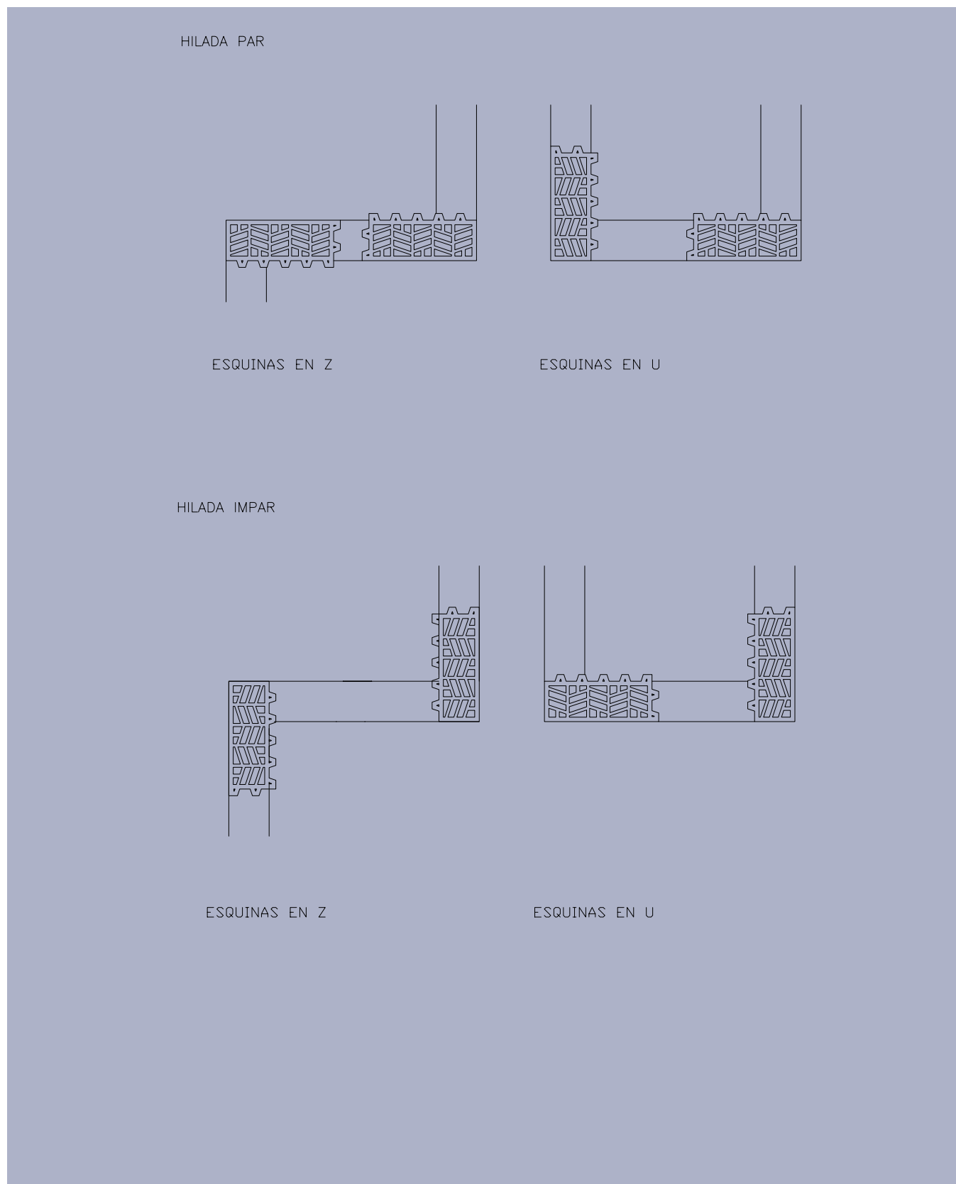
Figura 49: Ejecución de las esquinas. Replanteo con piezas de esquina.
